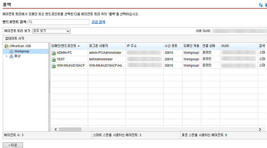
그림 2-8. 롤백 화면
