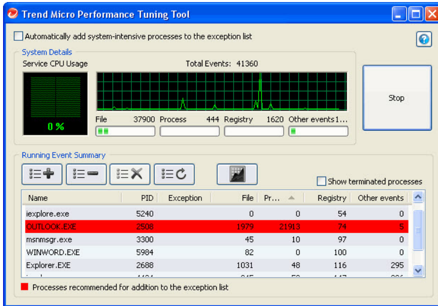
그림 15-1. 강조 표시된 시스템 집약적인 프로세스
