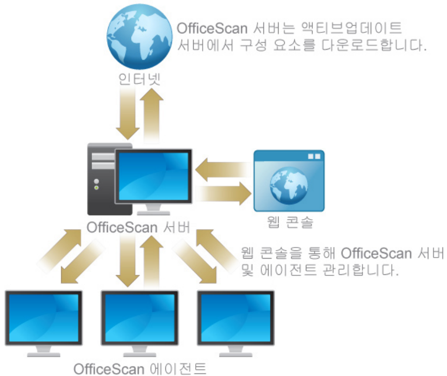
그림 1-1. OfficeScan 서버 작동 방식
