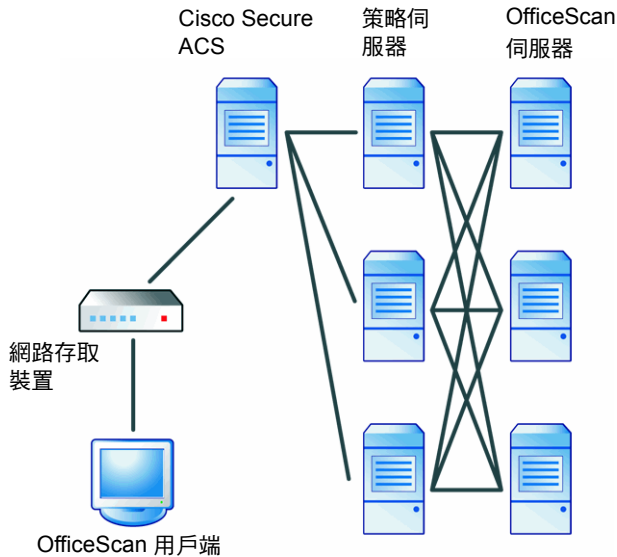
圖 15-3. 多部 Policy Server 和 OfficeScan 伺服器之間的關係
