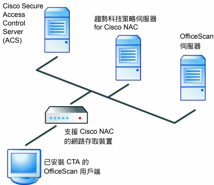
圖 15-1. 基本 Cisco NAC 架構
