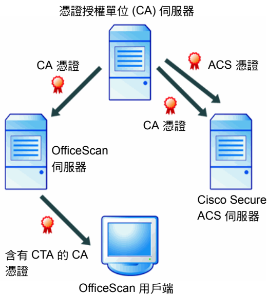
圖 15-4. 建立和部署 ACS 和 CA 憑證
