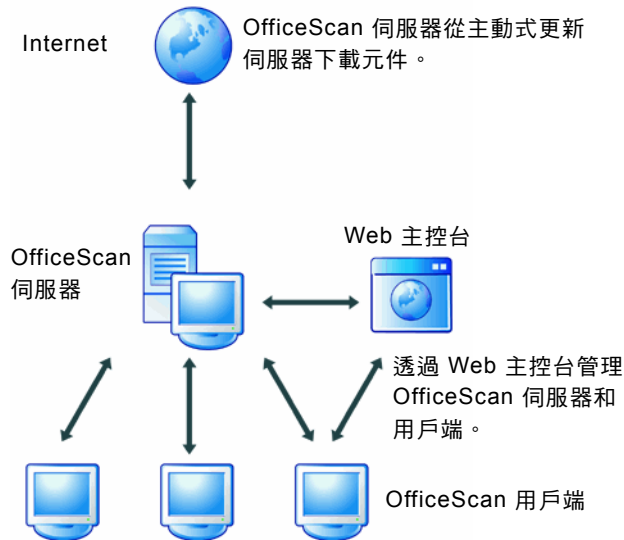
圖 1-1. OfficeScan 伺服器的運作方式
