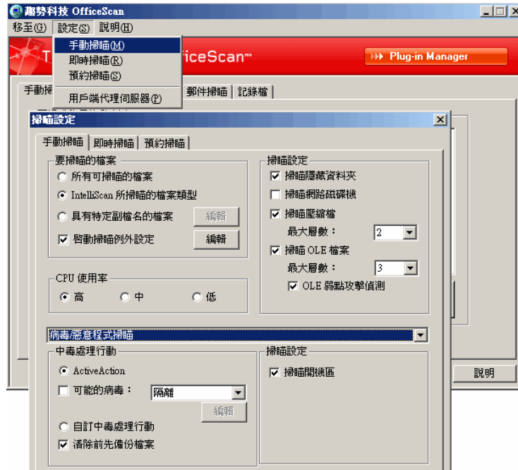
圖 6-1. 用戶端主控台上的掃瞄設定
