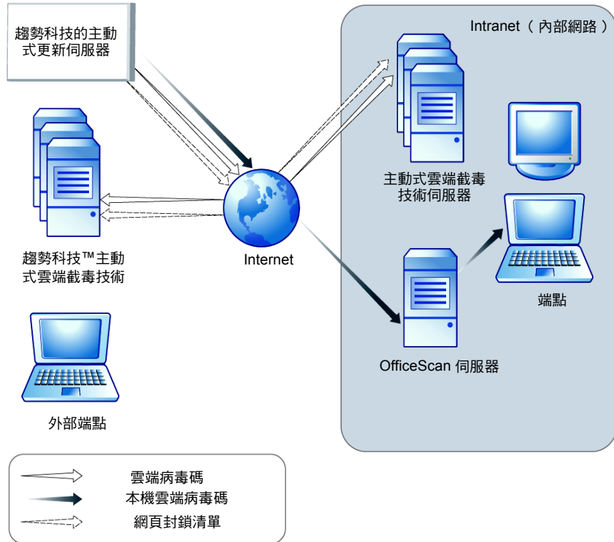
圖 3-1. 病毒碼更新程序
