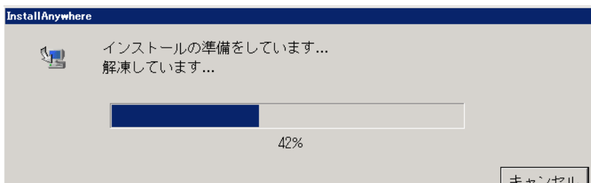
図 2-31. [InstallAnywhere] 画面
