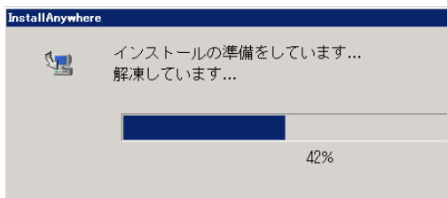
図 2-1. [InstallAnywhere] 画面
