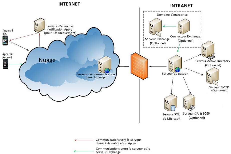
FIGURE 1-1. Modèle de sécurité renforcée avec le serveur de communication du nuage
