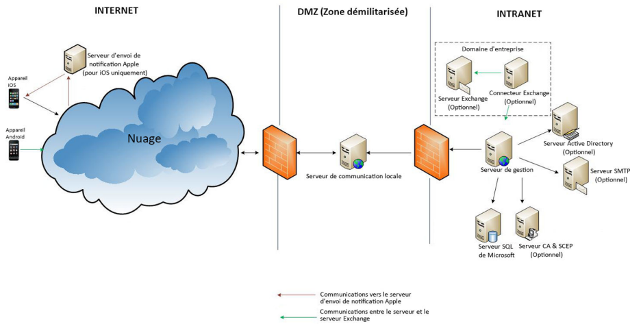
FIGURE 1-2. Modèle de sécurité renforcée avec serveur de communication local
