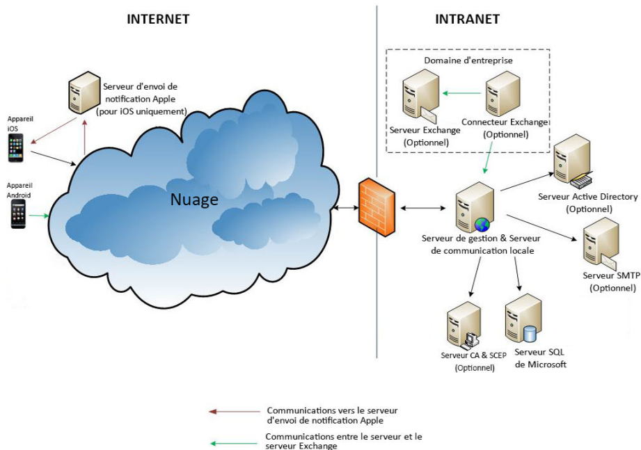
FIGURE 1-3. Modèle de sécurité de base
